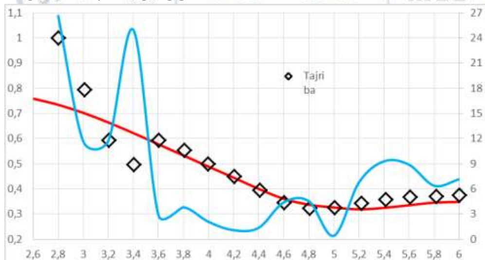
1-rasm. Nikuradze tajribasini analitik xisoblash grafigi
